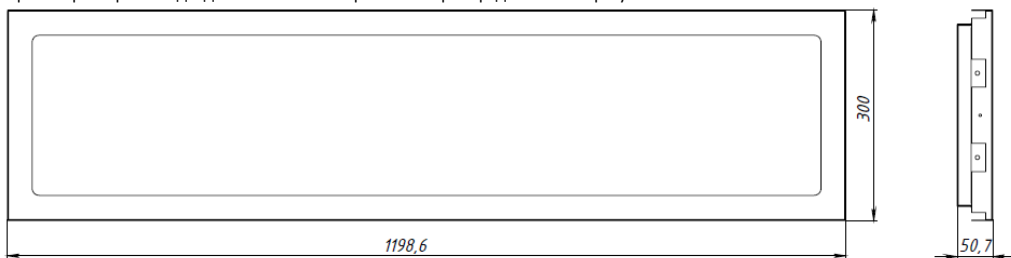
Рисунок 1 — Габаритные и установочные размеры светильника Geniled Office Clip-In 1200x300x60.
